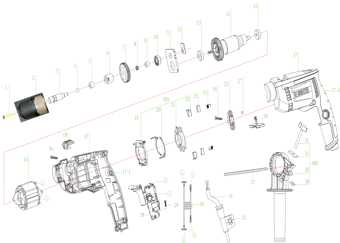
РИСУНОК А. АППАРАТ В РАЗБОРЕ
